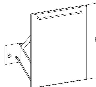
I Cassetto I per per cassetiera da 640 mm. Drawer I for unit 640 mm.
