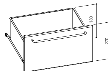
D Cassetto D per mobile da 500 mm. Drawer D for unit 500 mm.
