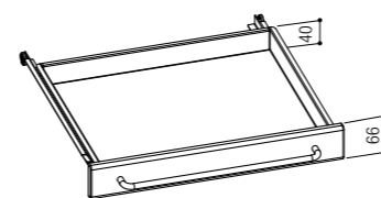
A Cassetto A per mobile da 500 mm. Drawer A for unit 500 mm.
