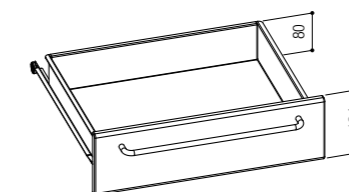
B Cassetto B per mobile da 500 mm. Drawer B for unit 500 mm.
