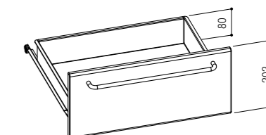
C Cassetto C per mobile da 500 mm. Drawer C for unit 500 mm.
